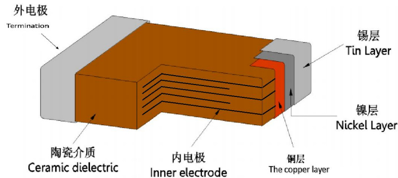
图 1 片式多层陶瓷电容器外形与内部结构 Figure 1 Dimension and Cross-section of MLCC
